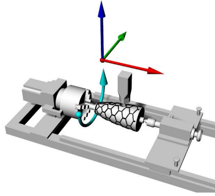
Görsel 4. Döner eksenli yazıcı ile form şekillendirme ( http://mkmra2.blogspot.com/2020/12/rotary-axis-ceramic-printing.html )
