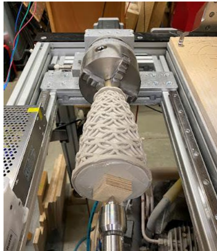
Görsel 6. Döner eksenli yazıcı ile form şekillendirme ( http://mkmra2.blogspot.com/2020/12/rotary-axis-ceramic-printing.html )
