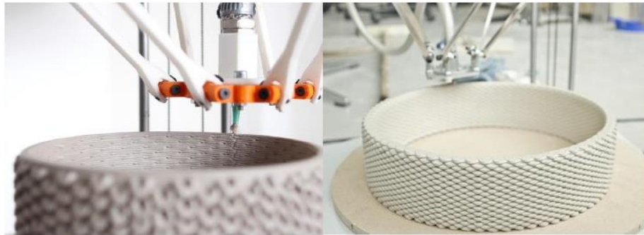
Görsel 2. FDM (harç yığıma) yazıcı ile form şekillendirme (Özgüven, 2015)
